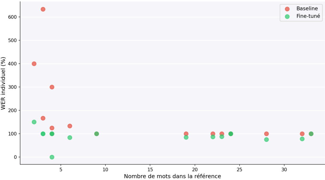
WER par audio selon la longueur de la transcription
