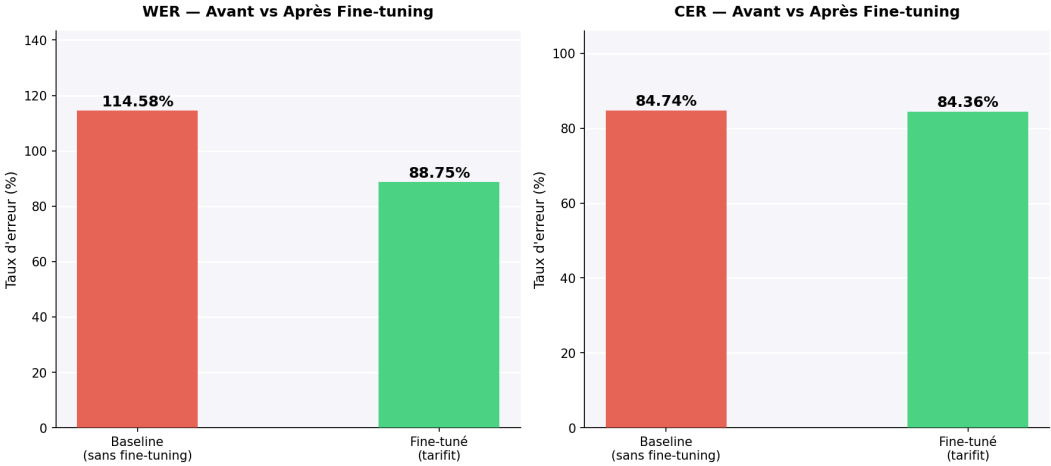
Fine-tuning Whisper-Small sur Tarifit Amélioration WER : 22.6% | Amélioration CER : 0.5%
