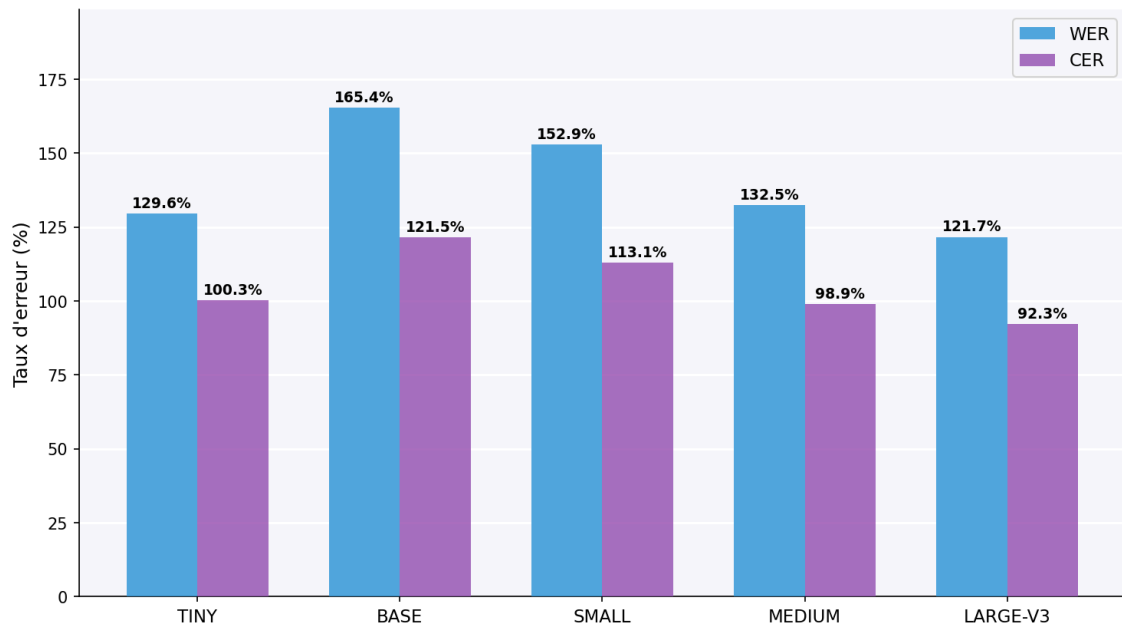
Comparaison WER/CER — Tous les modèles Whisper (Baseline Tarifit)
